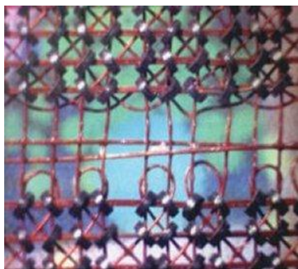
Memoria a nuclei di ferrite dell'ELEA 6001 - Anni '60
